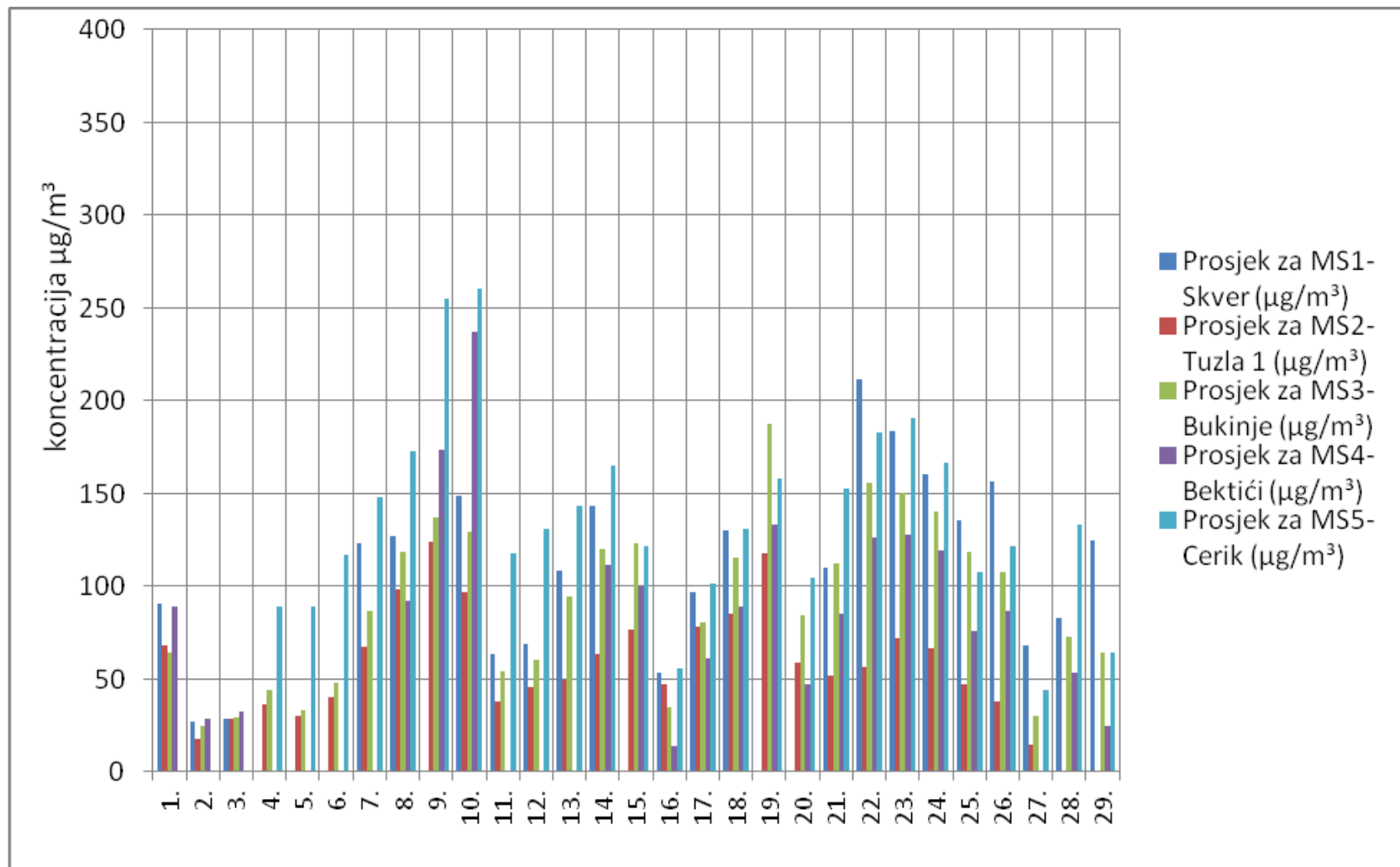
Slika 5. Grafički prikaz prosječnih dnevnih vrijednosti lebdećih čestica (PM 2.5 ) za mjesec februar/veljača 2012. godine
