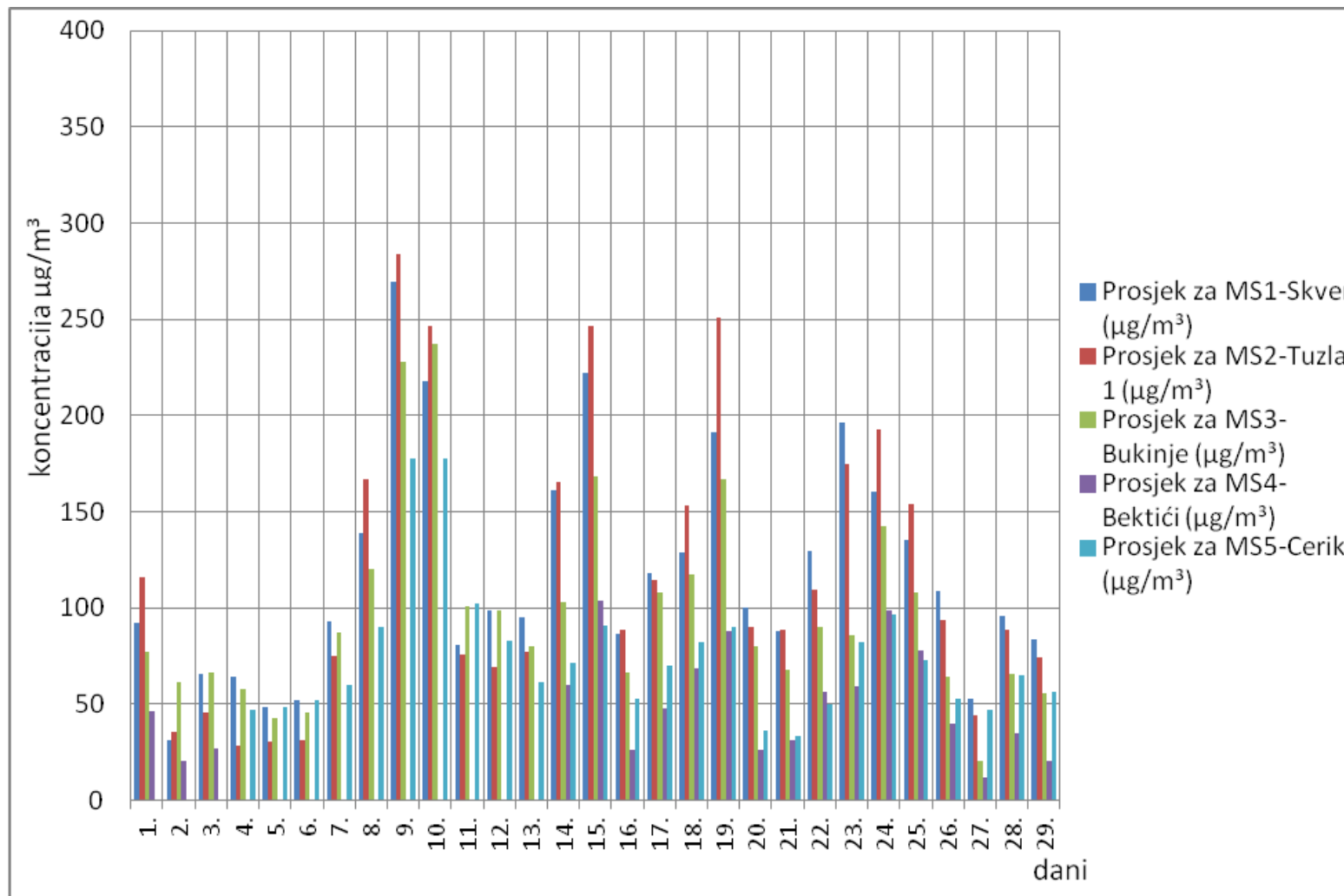
Slika 1. Grafički prikaz prosječnih dnevnih vrijednosti sumpordioksida (SO 2 ) za mjesec februar/veljača 2012. godine
