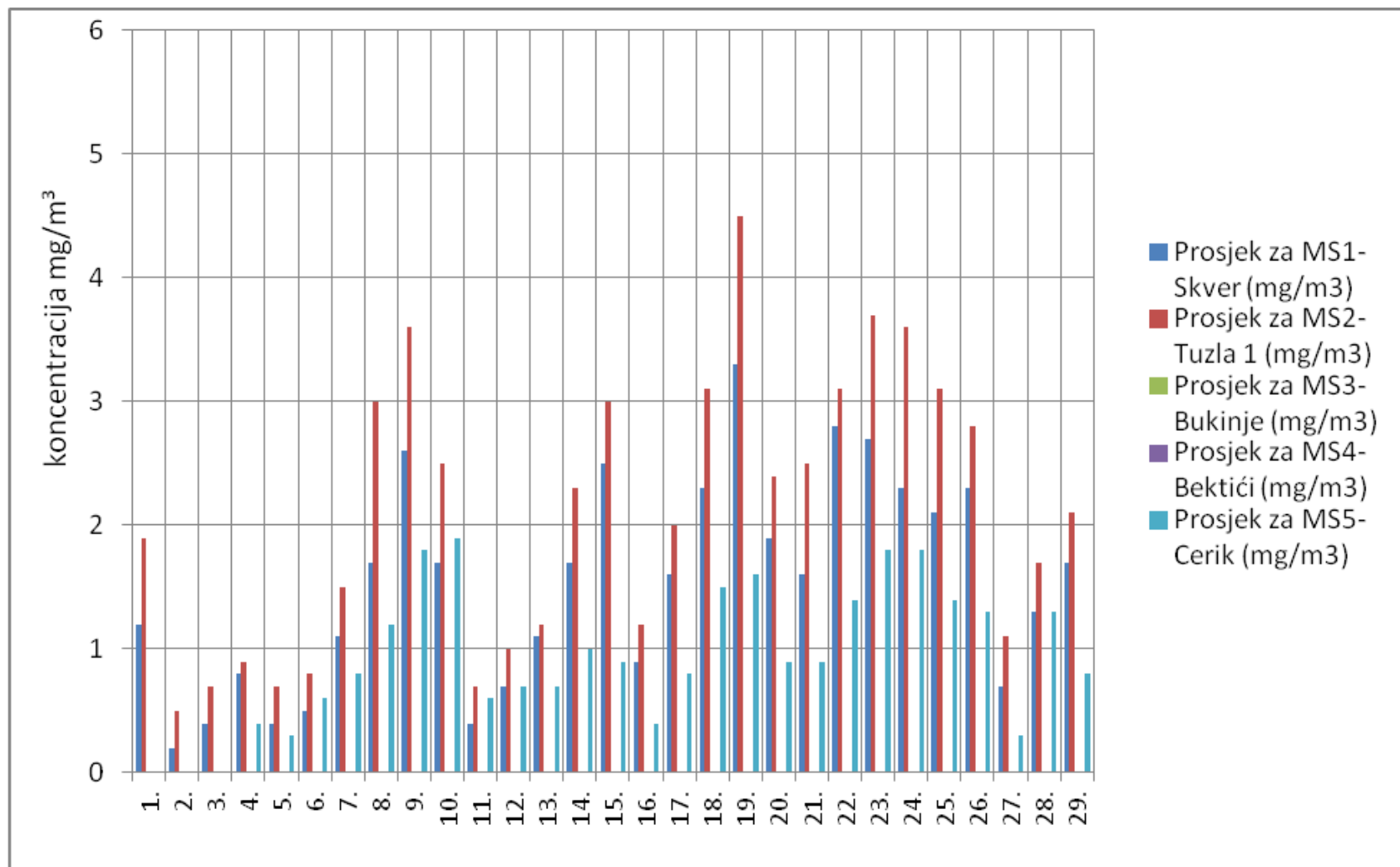
Slika 3. Grafički prikaz prosječnih dnevnih vrijednosti ugljenmonoksida (CO) za mjesec februar/veljača 2012. godine
