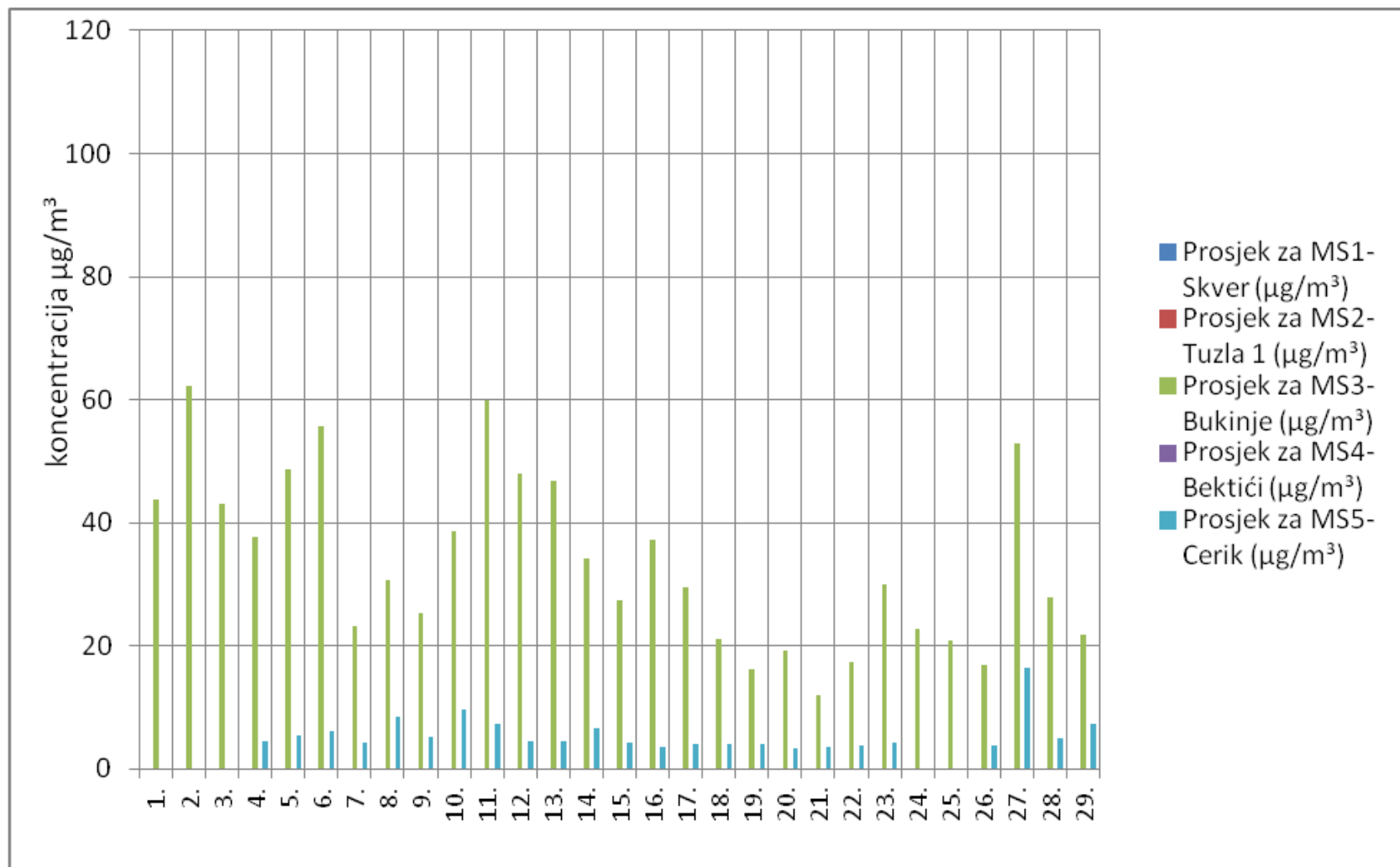
Slika 4. Grafički prikaz prosječnih dnevnih vrijednosti ozona ( \text{O}_3 ) za mjesec februar/veljača 2012. godine
