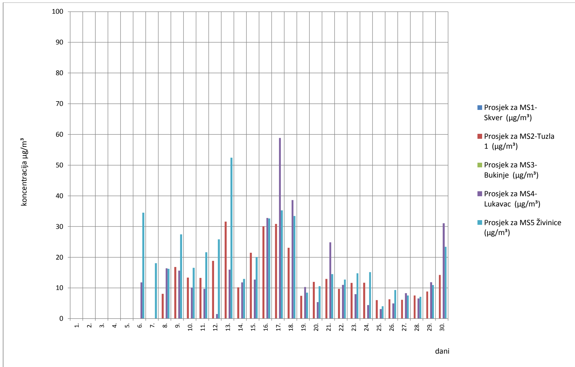
Slika 4. Grafički prikaz prosječnih dnevnih vrijednosti ugljenmonoksida ( \text{O}_3 ) za mjesec novembar/studeni 2019. godine
