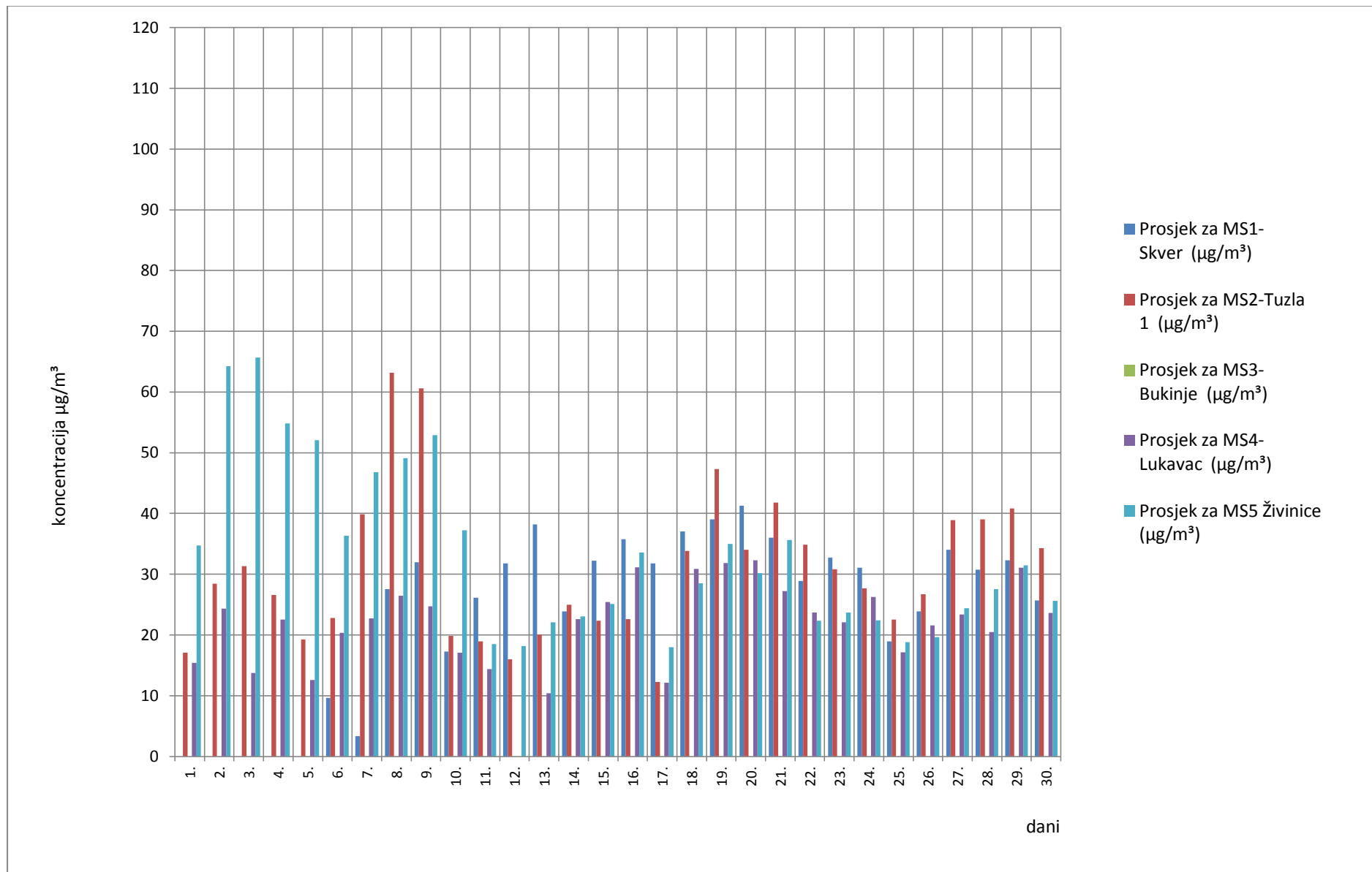
Slika 2. Grafički prikaz prosječnih dnevnih vrijednosti azotdioksida ( \text{NO}_2 ) za mjesec novembar/studeni 2019. godine
