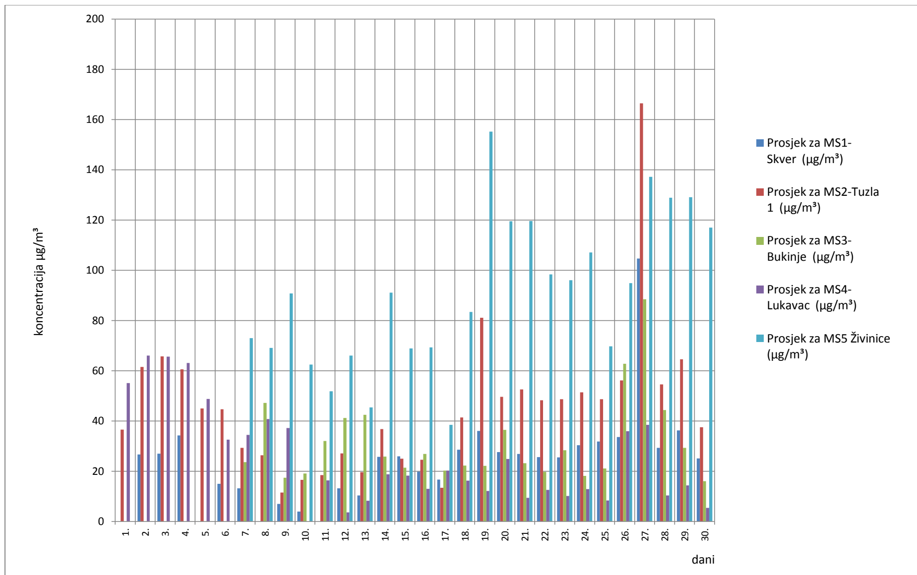
Slika 1. Grafički prikaz prosječnih dnevnih vrijednosti sumpordioksida (SO 2 ) za mjesec novembar/studeni 2019. godine
