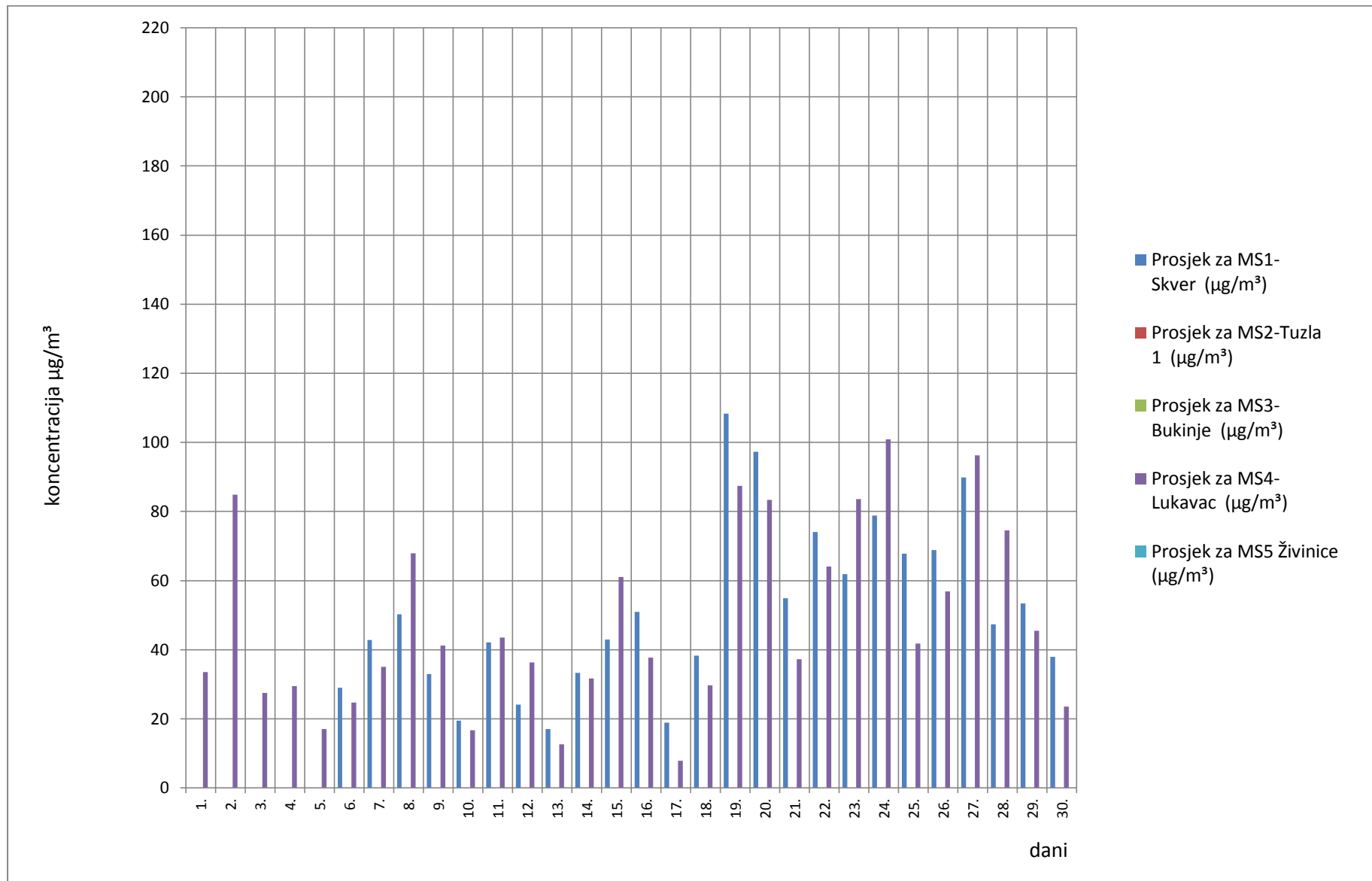
Slika 5. Grafički prikaz prosječnih dnevnih vrijednosti suspendovanih čestica (PM 2,5 ) za mjesec novembar/studeni 2019. godine
