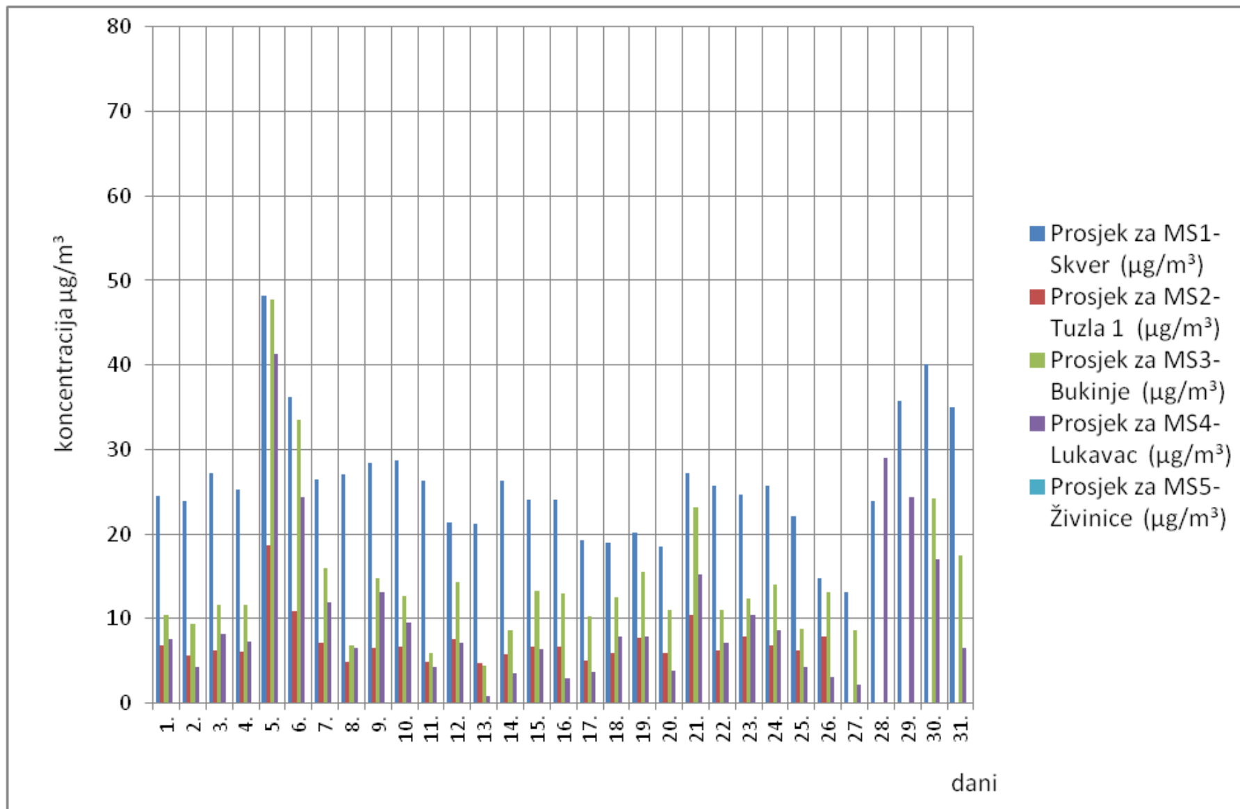
Slika 4. Grafički prikaz prosječnih dnevnih vrijednosti ozona ( \text{O}_3 ) za mjesec januar/siječanj 2020. godine
