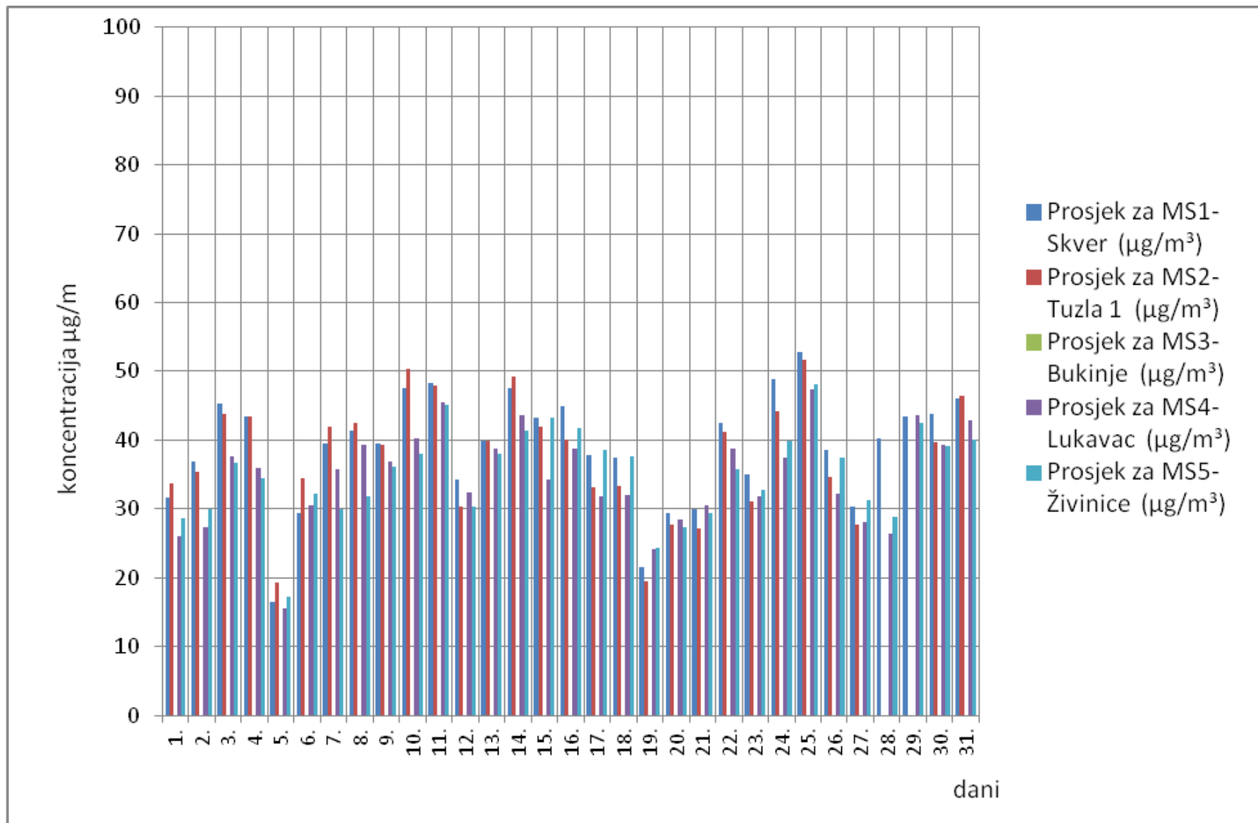
Slika 2. Grafički prikaz prosječnih dnevnih vrijednosti azotdioksida (NO 2 ) za mjesec januar/siječanj 2020. godine
