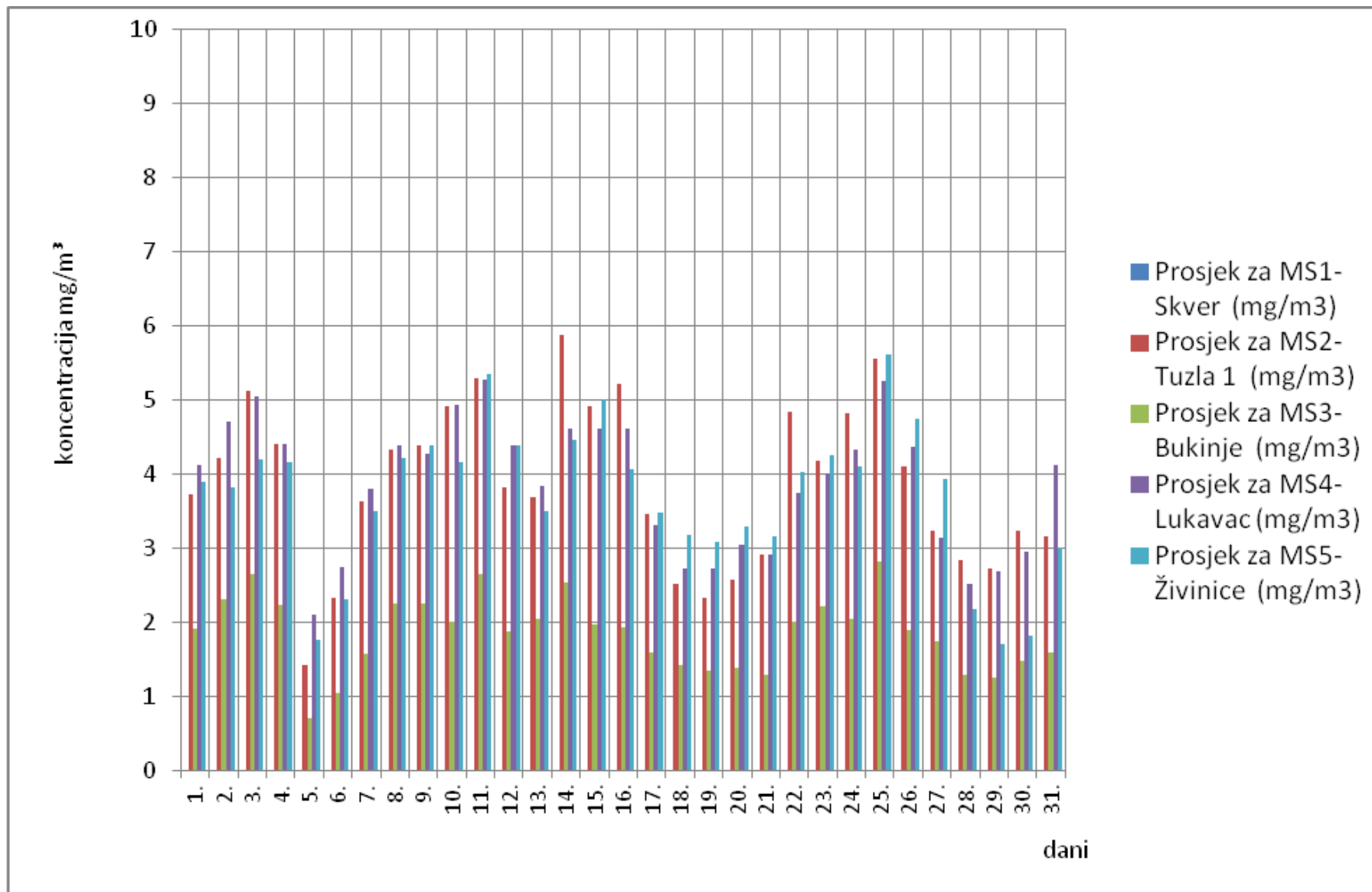
Slika 3. Grafički prikaz prosječnih dnevnih vrijednosti ugljenmonoksida (CO) za mjesec januar/siječanj 2020. godine
