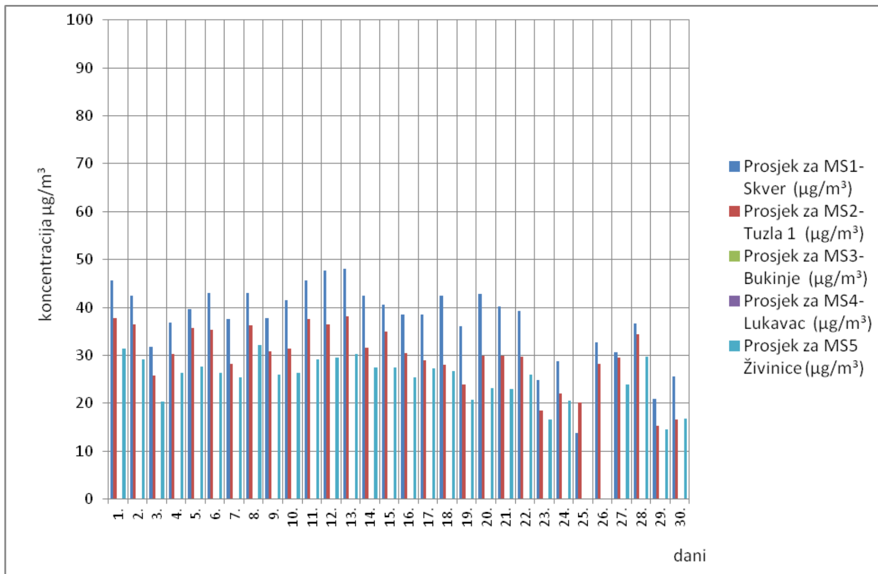
Slika 4. Grafički prikaz prosječnih dnevnih vrijednosti ozona ( \text{O}_3 ) za mjesec septembar/rujan 2020. godine
