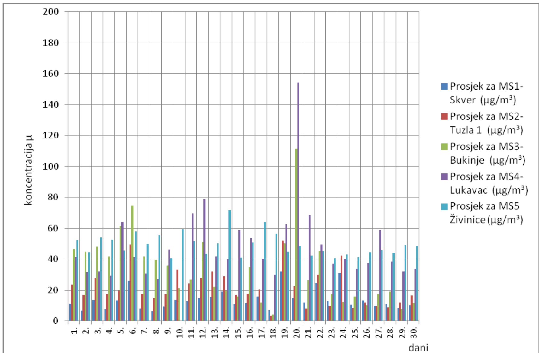
Slika 1. Grafički prikaz prosječnih dnevnih vrijednosti sumpordioksida (SO 2 ) za mjesec septembar/rujan 2020. godine
