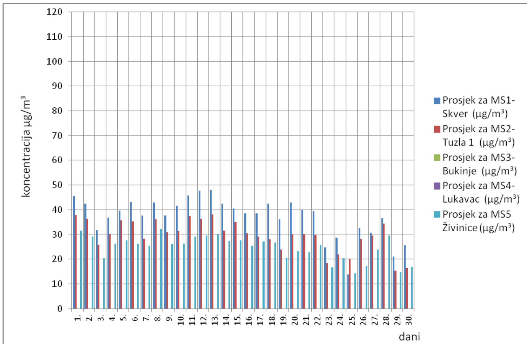
Slika 5. Grafički prikaz prosječnih dnevnih vrijednosti suspendovanih čestica (PM 2,5 ) za mjesec septembar/rujan 2020. godine
