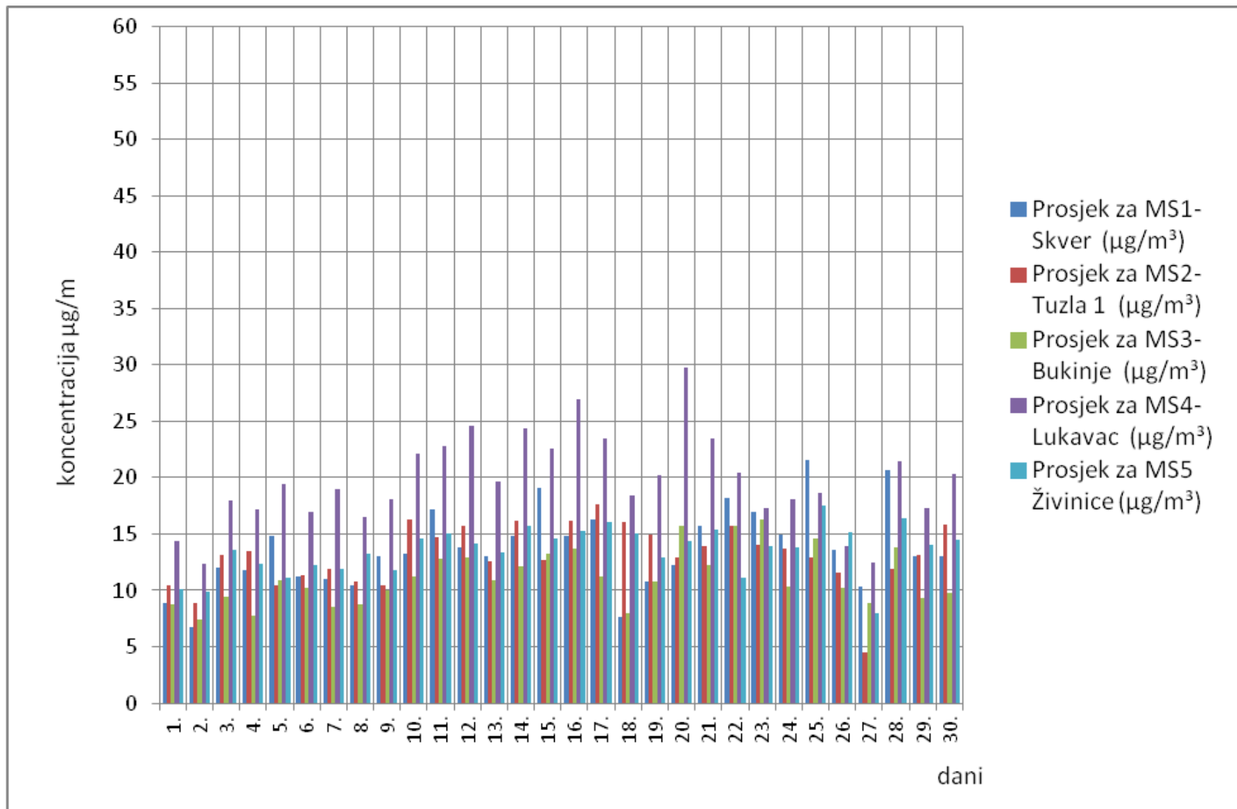
Slika 2. Grafički prikaz prosječnih dnevnih vrijednosti azotdioksida (NO 2 ) za mjesec septembar/rujan 2020. godine
